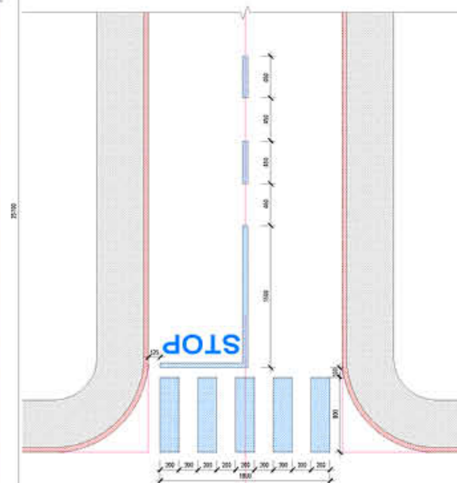
ŠÍRKA KOMUNIKÁCIE M 1:25
