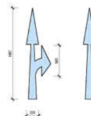
DOPRAVNÉ ZNAČENIE M 1:25
